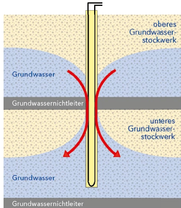
Abb. 8: Unzureichend abgedichtete Erdwärmebohrung. Grundwasser strömt in diesem Beispiel von einem höheren in ein tieferes Grundwasserstockwerk. Bei einem höheren Druckniveau im tieferen Stockwerk (gespanntes Grundwasser) kann auch ein Aufstieg des Grundwassers in das obere Stockwerk oder sogar bis zur Geländeoberfläche stattfinden.
