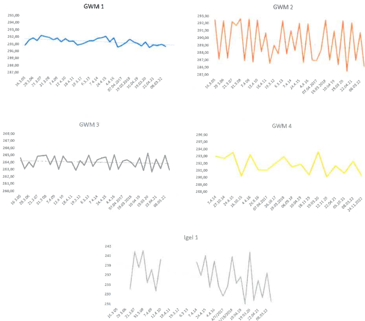
Abbildung 3: Vergleich der Grundwasserstände 2005 - 2022
