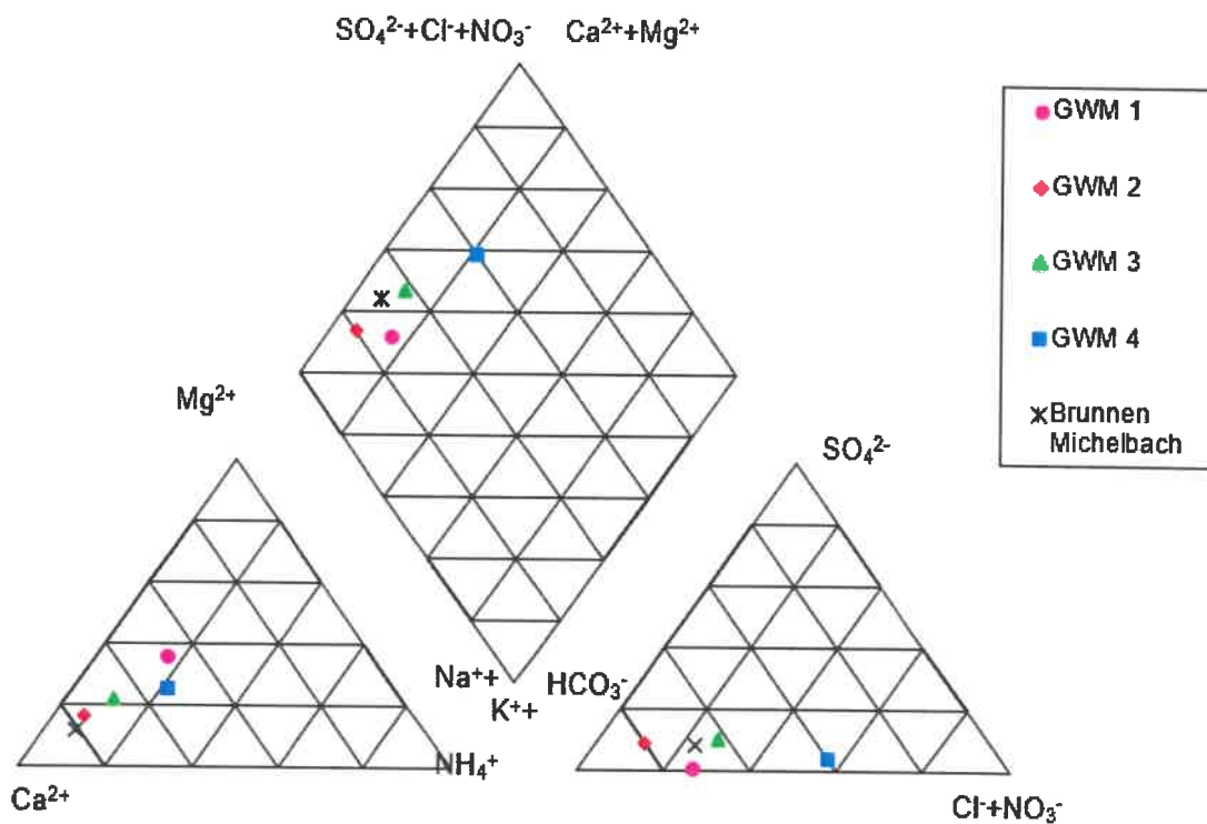
Abbildung 4: Darstellung der Ionenverhältnisse im Piper-Diagramm für den 24.11.2022 - Bereich ehemaliger Gemeindepfandplatz Michelbach
