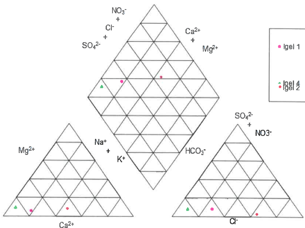
Abbildung 5: Darstellung der Ionenverhältnisse im Piper-Diagramm für den 24.11.2022 – Bereich Bauschutt-ablagerung Igelpfuhl
