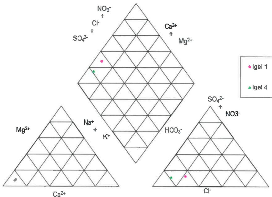
Abbildung 4: Darstellung der Ionenverhaltnisse im Piper-Diagramm fur den 12.11.2020 – Bereich Bauschuttanlage Igelpfuhl
