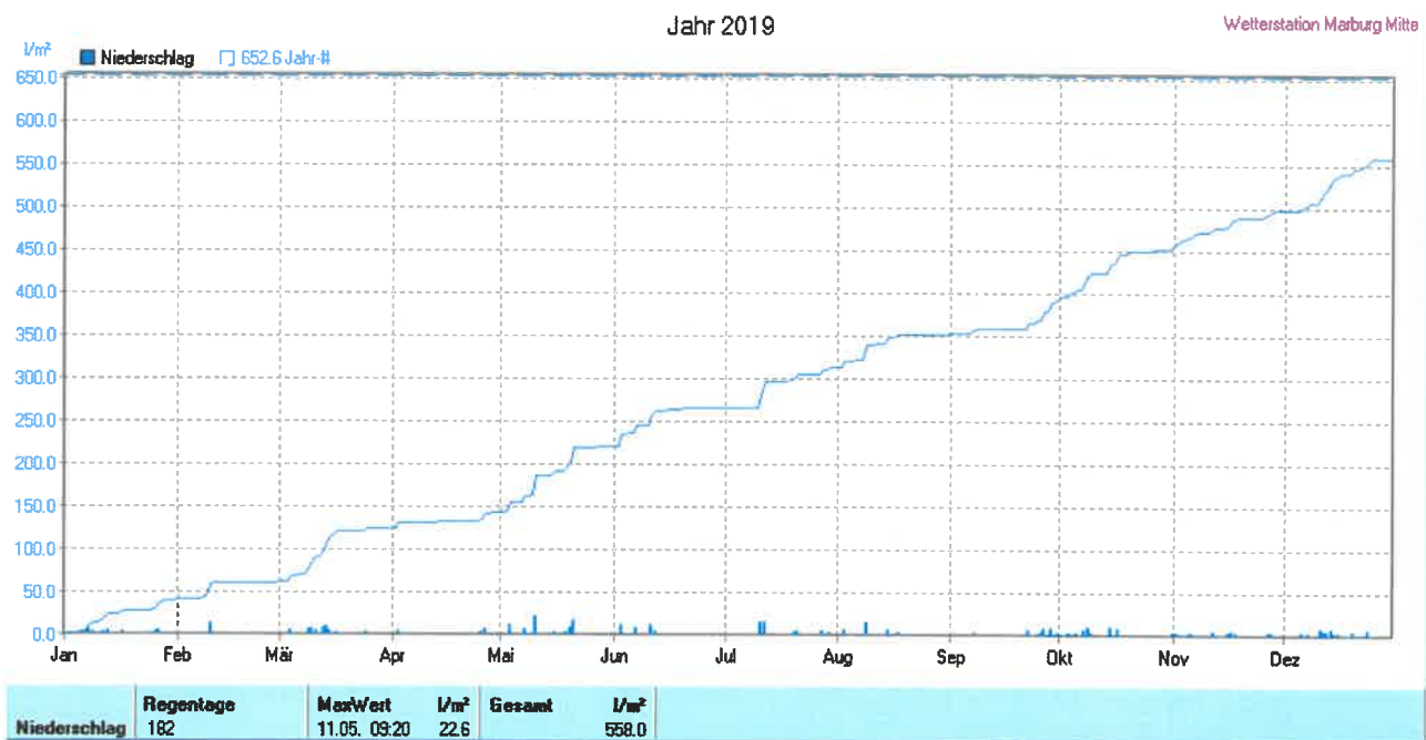
Abbildung 1: Jahresverlauf der Niederschläge 2019 für die Wetterstation Marburg-Mitte (Quelle: www.wettereule.de )
