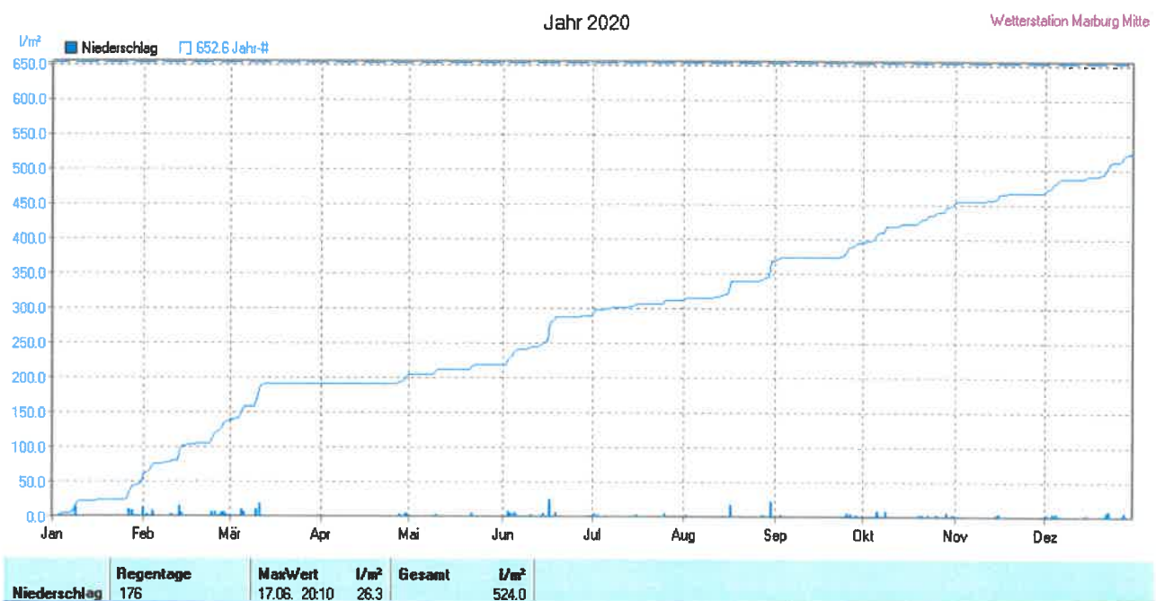
Abbildung 2: Jahresverlauf der Niederschläge 2020 für die Wetterstation Marburg-Mitte (Quelle: www.wettereule.de )
