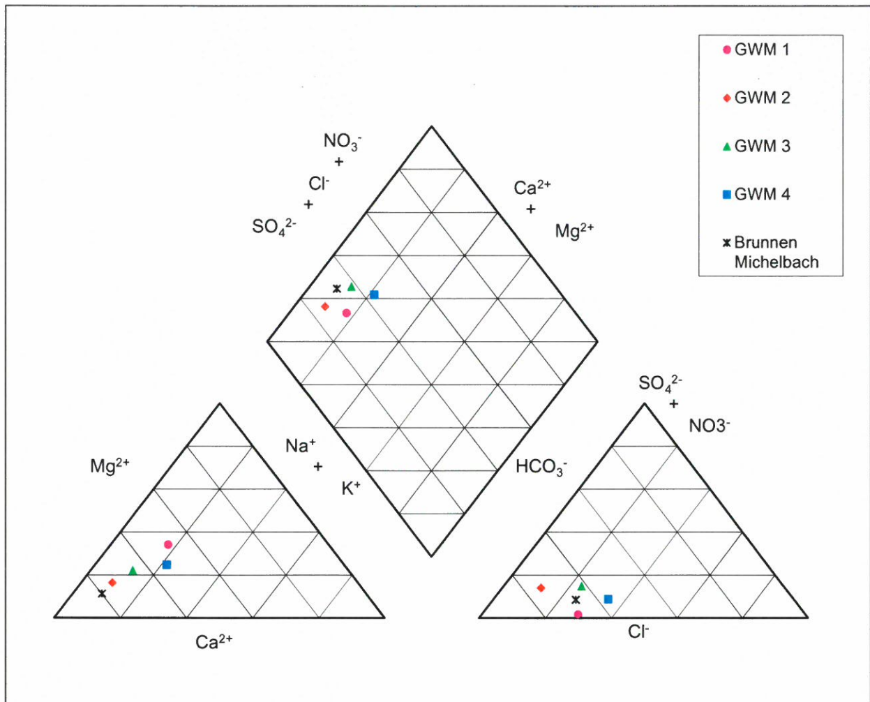
Abbildung 1: Darstellung der Ionenverhältnisse im Piper-Diagramm für den 07.04.2014
